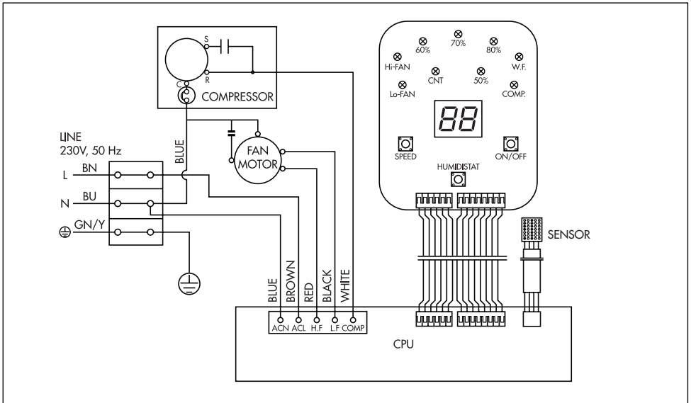
D850E / D950E wiring diagram
