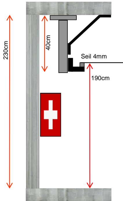
Deckenmontage mit Konsole mit Strebe:
