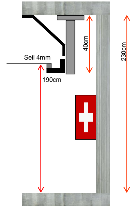
Deckenmontage mit Konsole mit Strebe:
