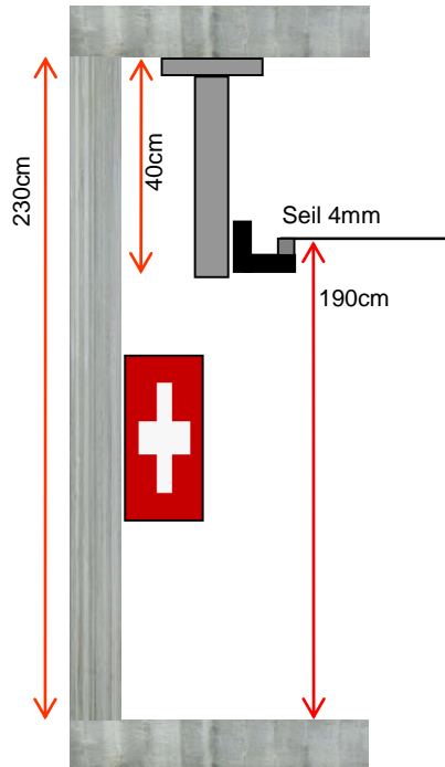
Deckenmontage mit Konsole:
