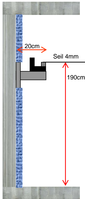
Wandmontage mit Konsole unter Isolation:
