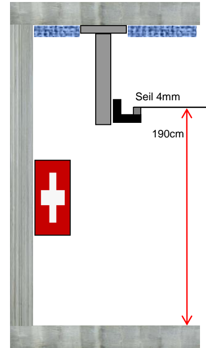
Deckenmontage mit Konsole unter Isolation:
