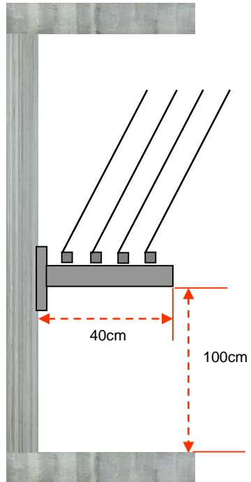
Juniorleine mit Konsole:
