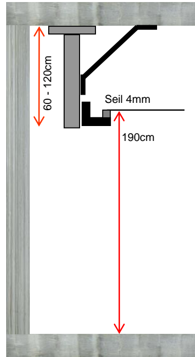
Deckenmontage mit Konsole und Strebe:
