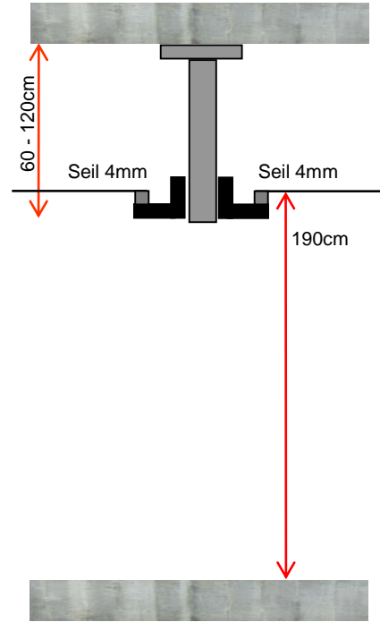
Deckenmontage mit Mittel-Konsole:
