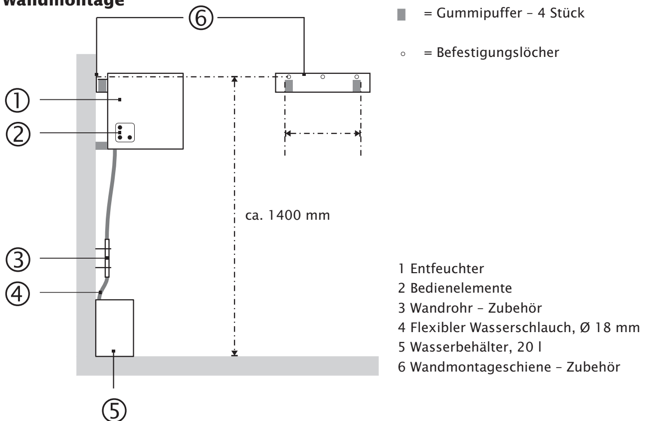
Abbildung 3 Wandmontage
